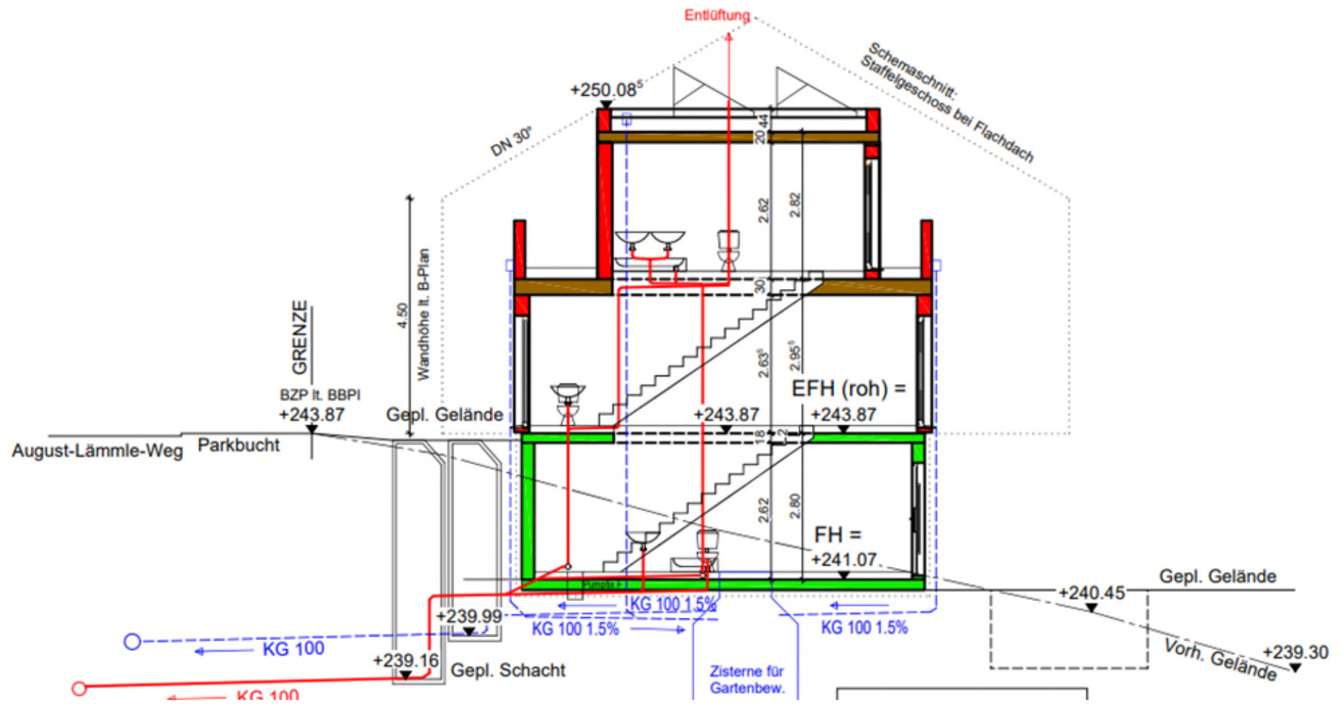
Schnitt A-A
